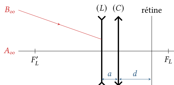
Figure 2 – Un œil myope et un verre de lunettes.
