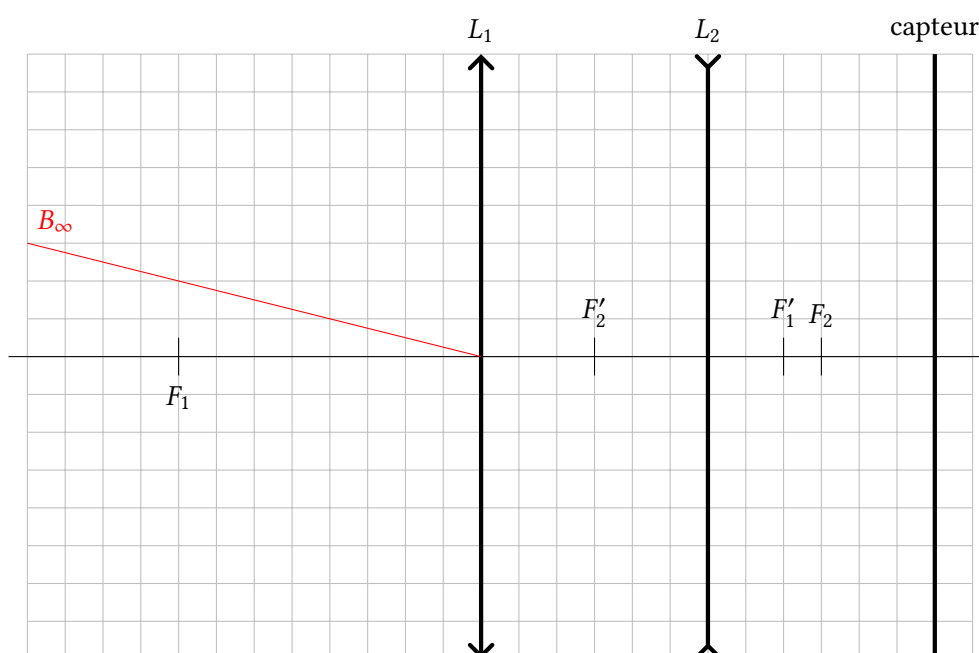
Figure 6 – Marche des rayons dans l'instrument.
