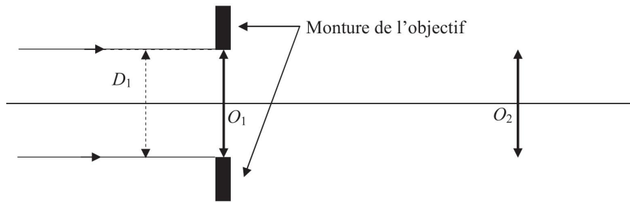
Figure 8 – Diaphragme d'ouverture d'une lunette astronomique.
