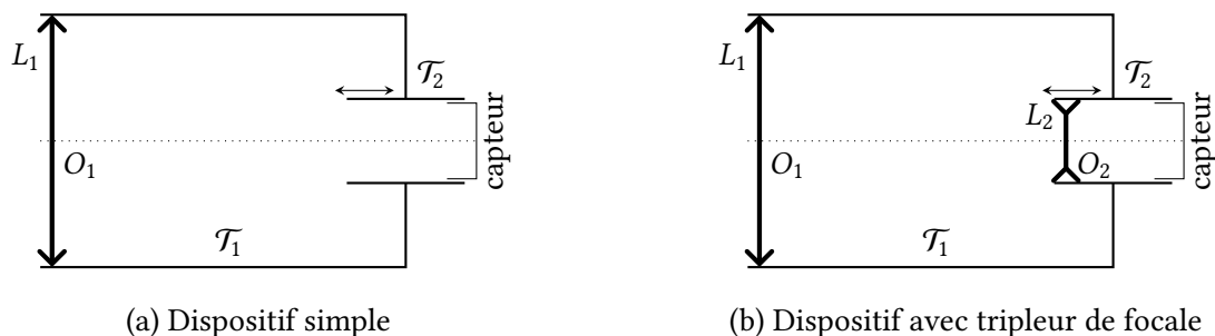
Figure 5 – Dispositif de photographie de Jupiter.
