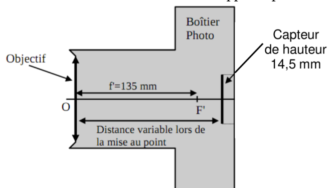
Document 2 : modélisation de l'appareil photo.
