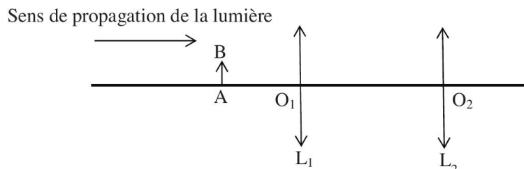
Figure 4 – Schéma du microscope optique classique.
