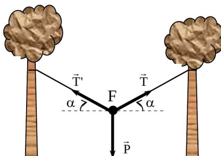
Figure 5 – Un point matériel en train de faire la sieste dans son hamac.
