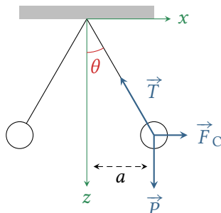
Figure 3 – Pendule électrostatique.
