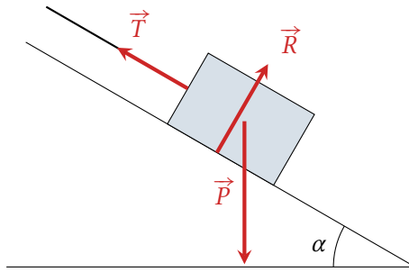
Figure 2 – Schéma des forces subies par le glaçon.
